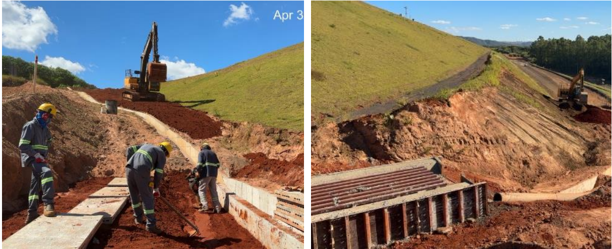
Figura 80 – Reaterro dos canais de drenagem e concretagem de travessia.
