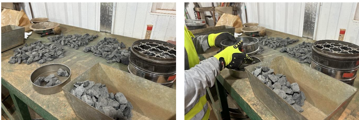
Figura 90 – Controle de qualidade e especificações realizado pela fiscalização – Ensaio de granulometria no enrocamento recebido.
