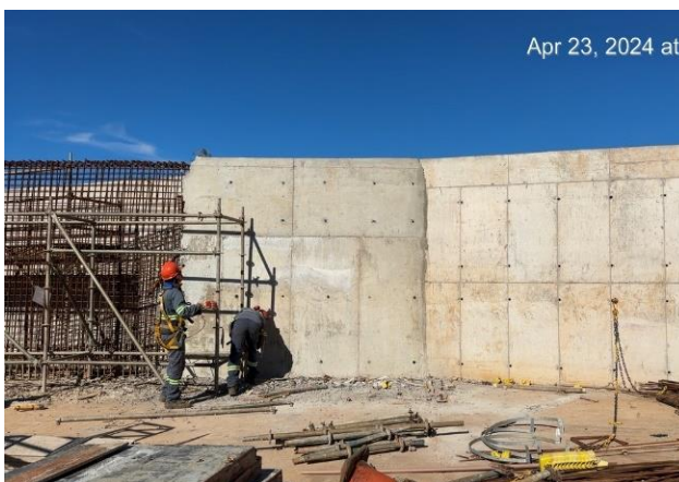
Figura 19 – Desforma das paredes da transição no canal rápido.
