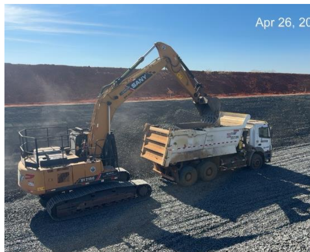
Figura 67 – Continuidade da aplicação da transição (areia, brita 0 e brita 3) sobre o revestimento em geomembrana.
