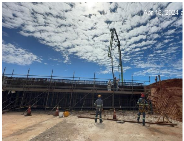
Figura 18 – Aplicação de concreto nas paredes da transição do canal rápido.
