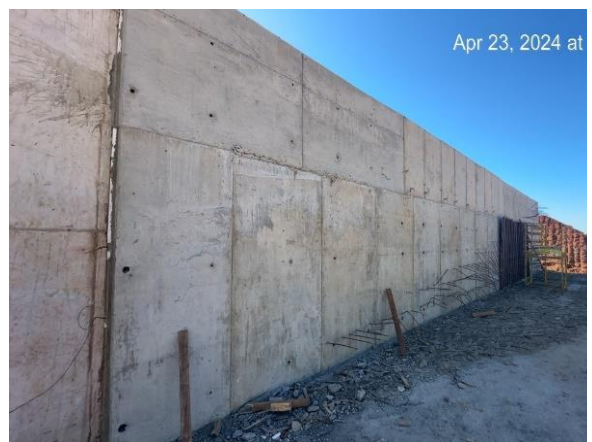
Figura 19 – Desforma das paredes da transição no canal rápido.
